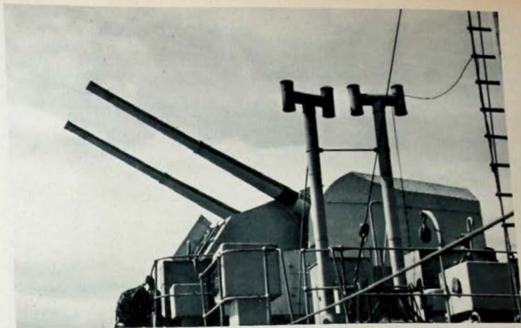
170. - Działo O.R.P. Orkan.
